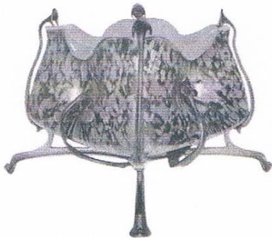
Delatte schaal
